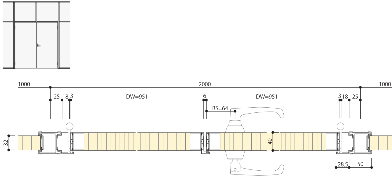
開戸（両開き）横断面図
