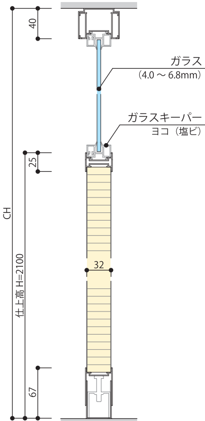
PG 縦断面図
