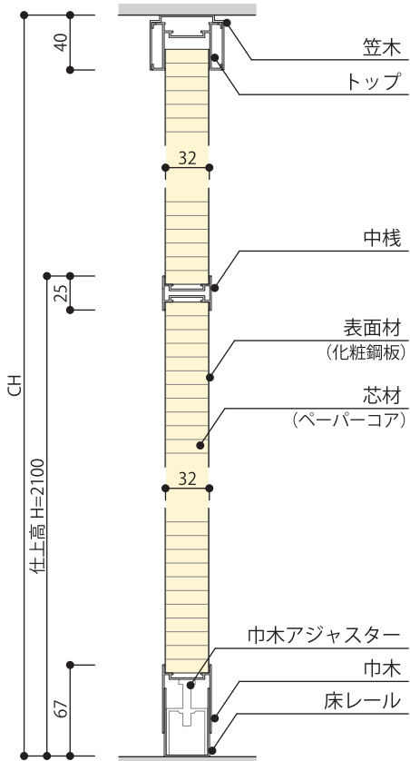
PP 縦断面図
