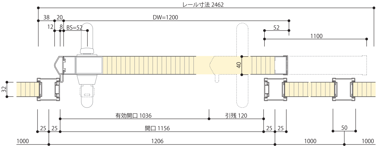
引戸（片引 オプション）横断面図
