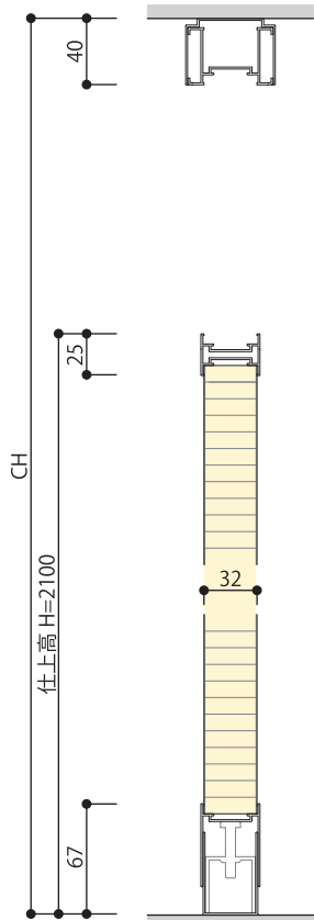
PO 縦断面図
