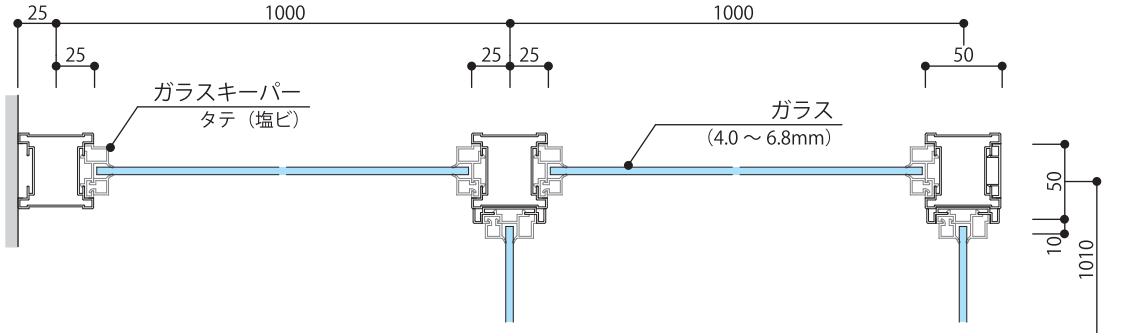
ガラス 横断面図
