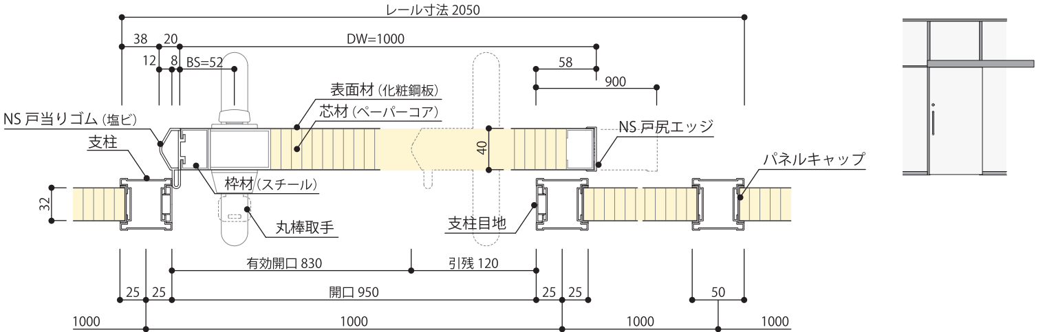
引戸（片引）横断面図
