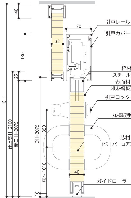
HDP 縦断面図
