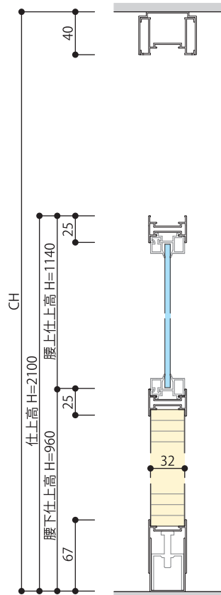
PGO 縦断面図
