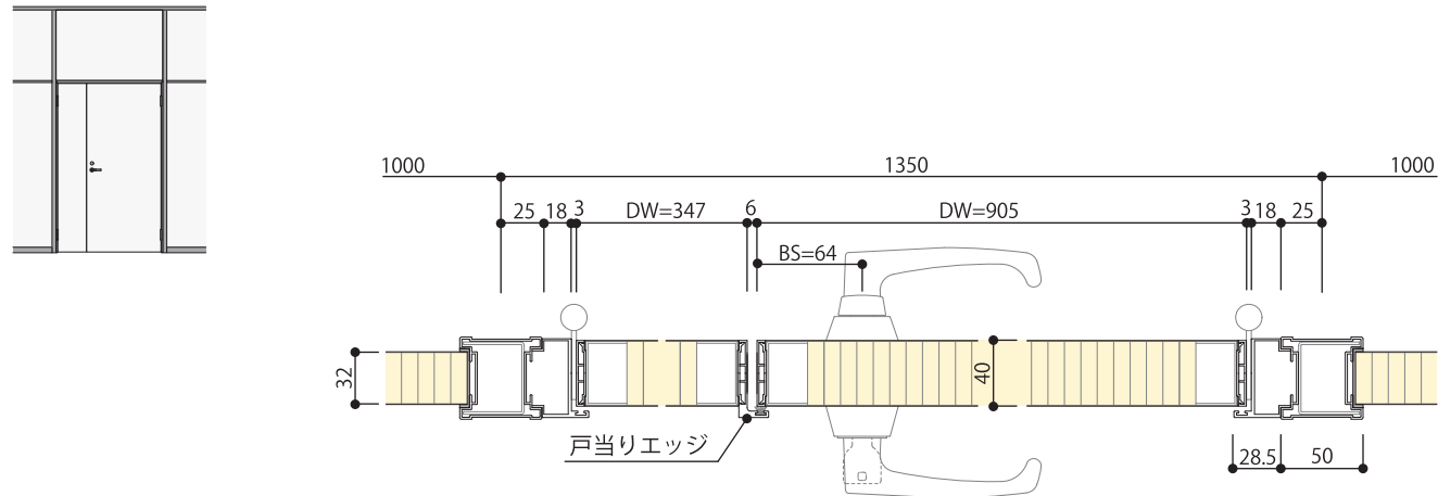
開戸（親子）横断面図
