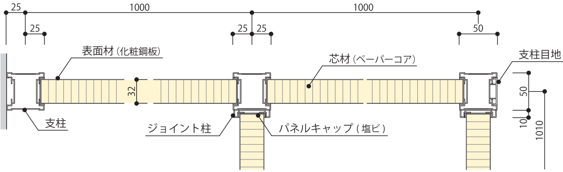
パネル 横断面図
