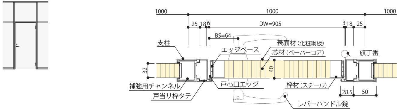
開戸（片開き）横断面図
