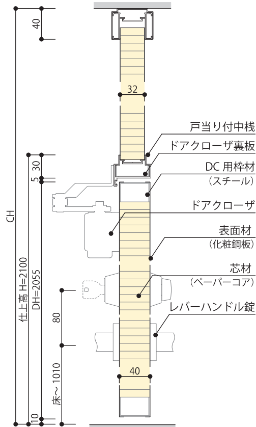
DP 縦断面図
