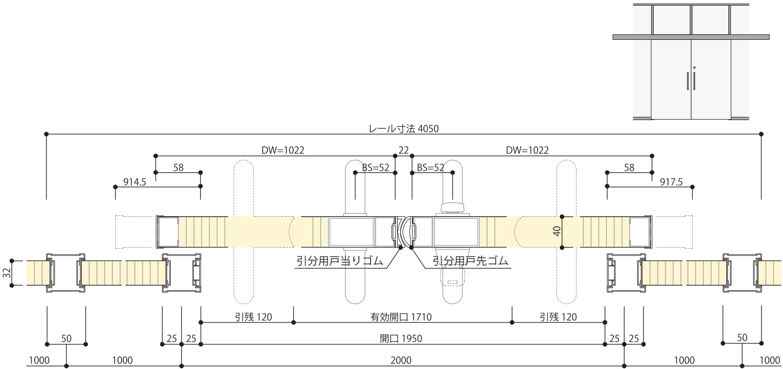
引戸（引分）横断面図
